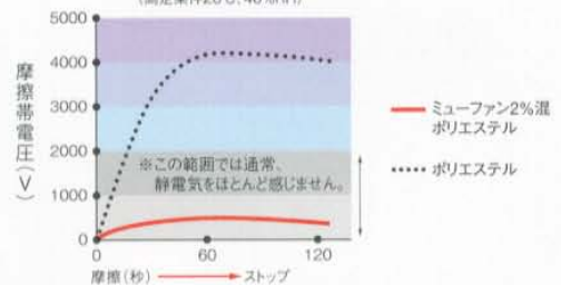
帯電防止機能テスト (測定条件20℃、40%RH)
